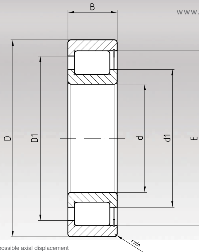
s 1 ) axial Verschiebeweg / possible axial displacement
